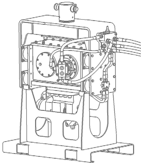
Рис. 12 Вибропогружатель на подставке
