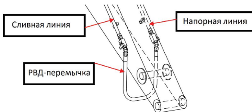
Рис. 9 Промывка трубопроводов при первичном подключении
