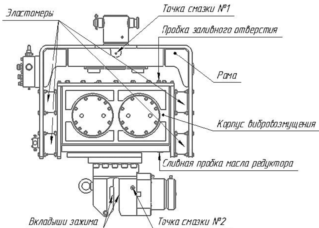
Рис. 5 Вибропогружатель
