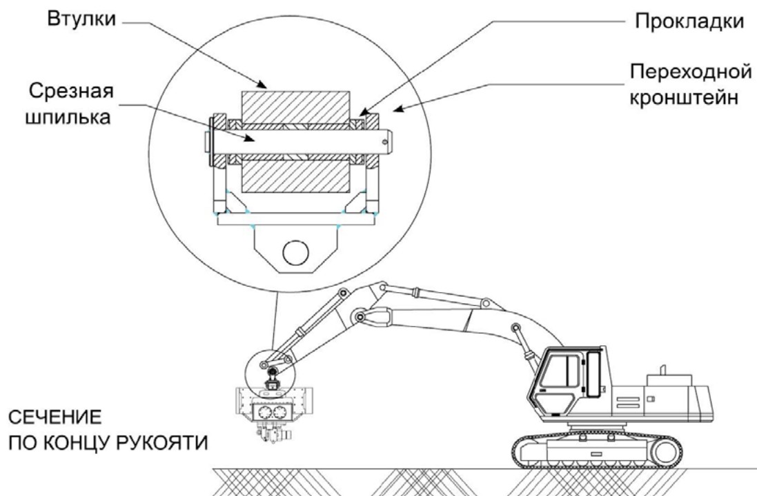
Рис. 6. Положение переходного адаптера на машине.
