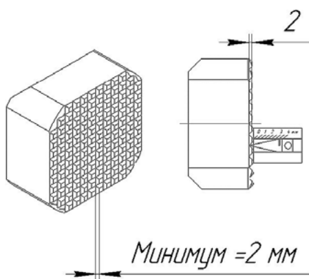
Рис. 4 Неподвижный вкладыш зажима.
